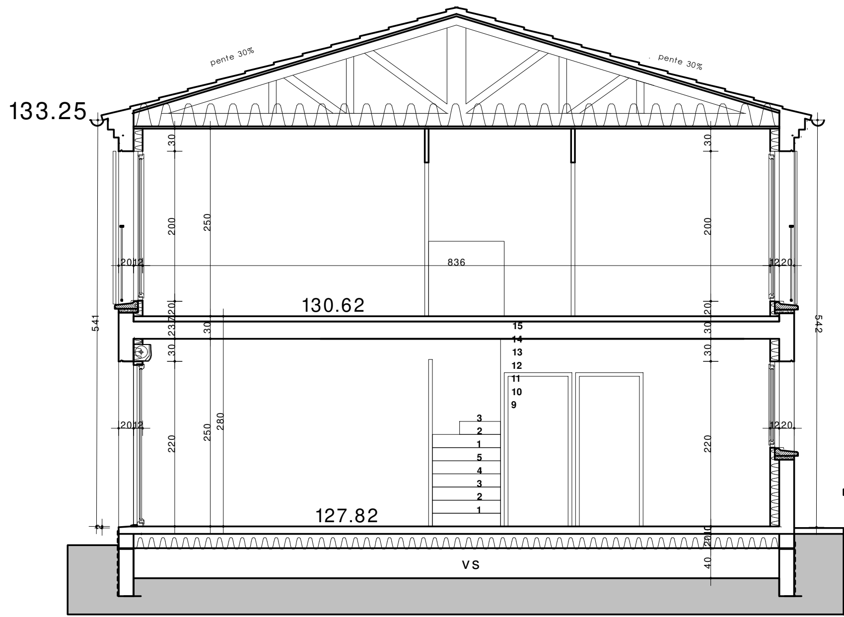
COUPES 1/50
