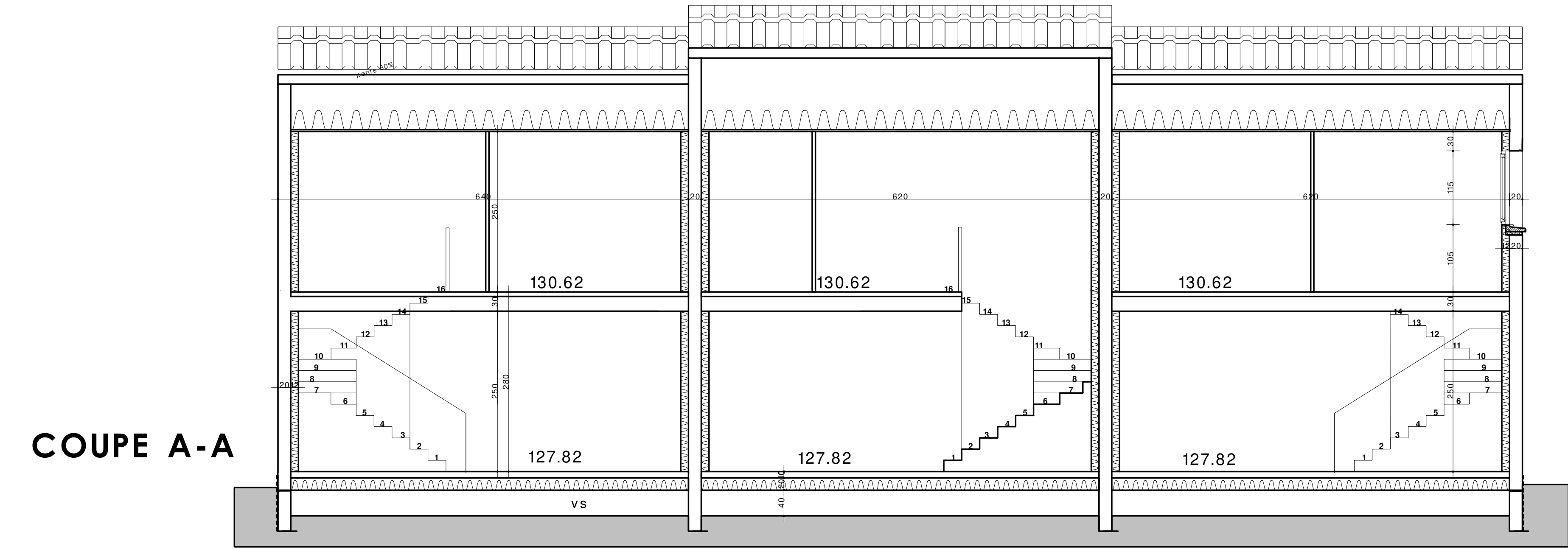
COUPES 1/50
